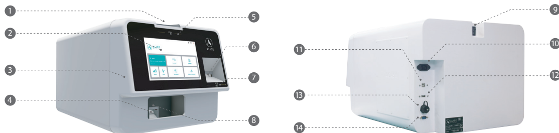
1.Entrada de moedas 2.Ecrã / touchscreen 3.Porta da máquina 4.Saída de moedas 5.Led indicativo de validador de moedas ativo 6.Entrada e saída de notas 7.Led indicativo de validador de notas ativo 8.Fechadura oculta para abertura da porta 9. Botão para ligação da máquina [ON/OFF] 10.Conetor cabo de alimentação 11.Conetor cabo OTG 12.Conetor cabo USB 13.Conetor Ethernet 14.Conetor de serviço RS232
